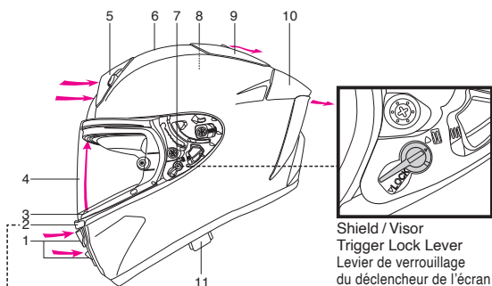
Upper Air Intake Entrée d'air supérieure
