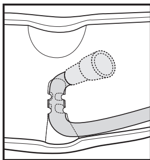
Εικόνα τοποθέτησης στοιχείου για τη λήψη υγρών Rysunek mocowania części układu nawadniania
