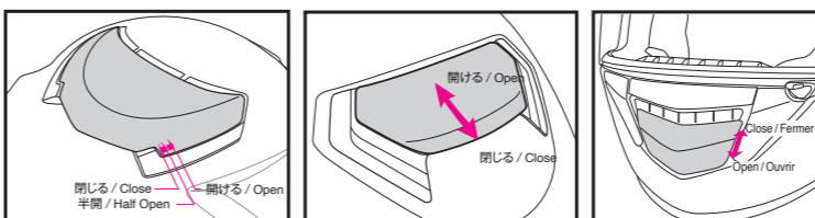
アッパー エア インテーク / Upper Air Intake トップ エア アウトレット / Top Air Outlet ロア エア インテーク / Lower Air Intake
